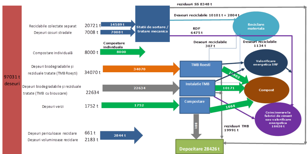
Figura 7.2. Schema fluxului de deșeurile municipale aferentă Alternativei "Unu" , anul 2025
