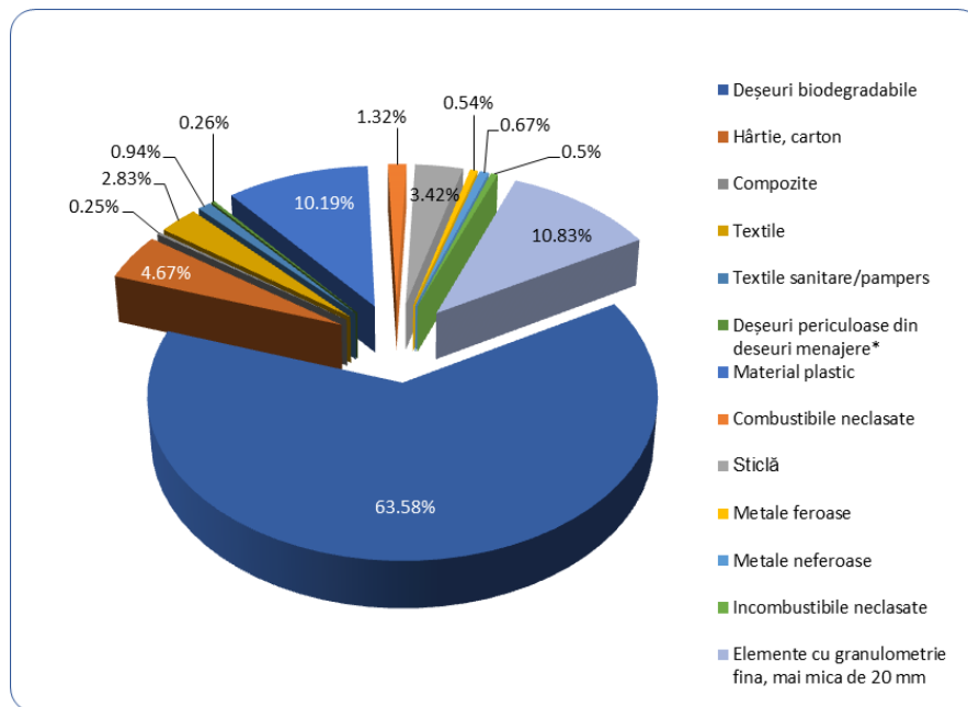
Figura 4.6. Compoziția deșeurilor menajere în mediul urban, în anul 2019
