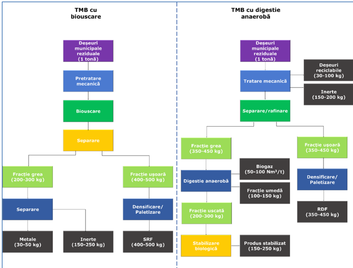
Figura 7.1. Fluxul tehnologic al instalațiilor TMB cu bioușcare și digestie anaerobă
