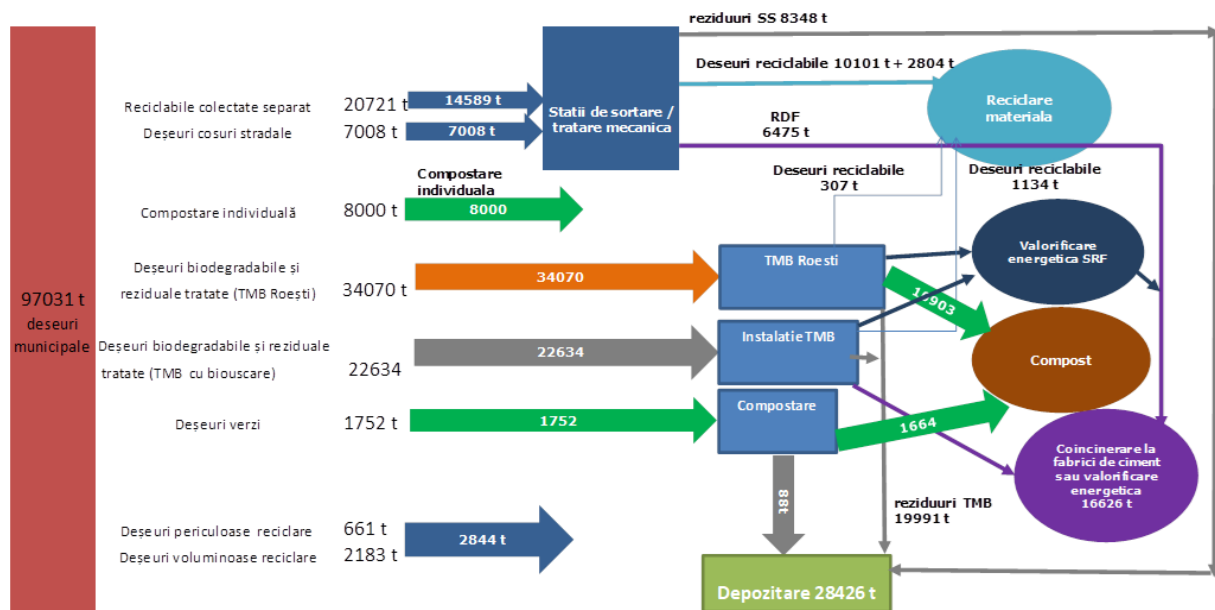
Figura 7.3. Schema fluxului de deșuri municipale aferentă Alternativa "Doi" , anul 2025
